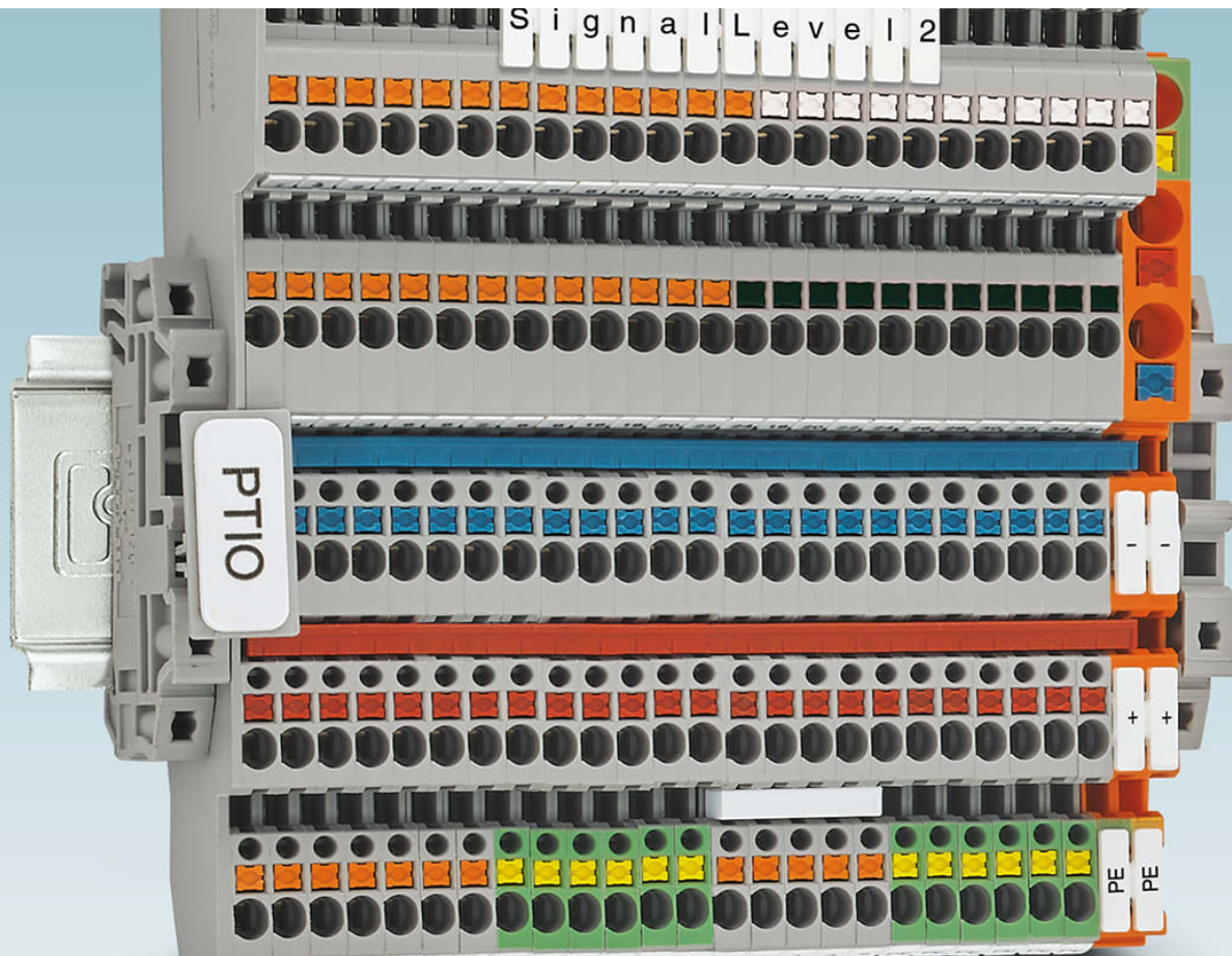
Givar-, ställdonsplintar PTIO 1,5/S/5 med dubbel signalgenomgång
